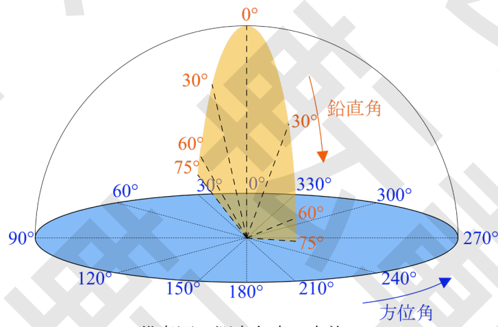
備考図 測定角度の定義
