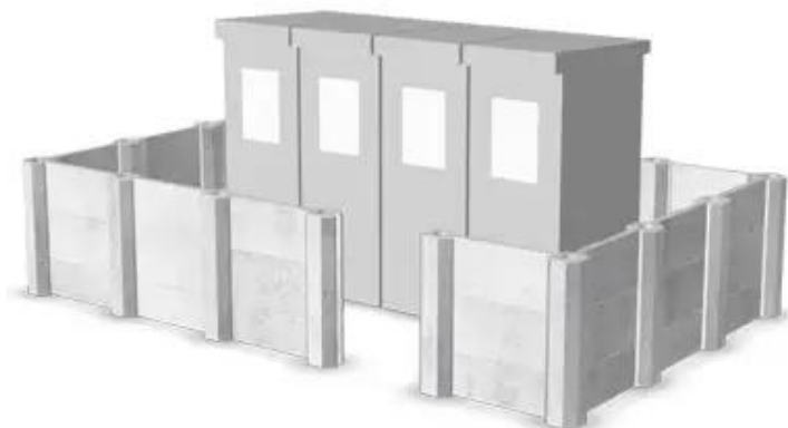
フェンスウォール®シリーズでできる止水工法施工図
