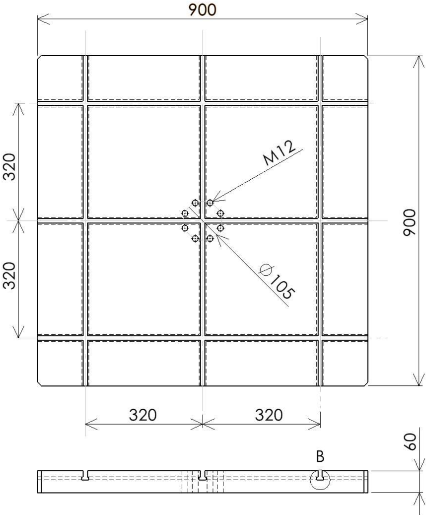
テーブル寸法
