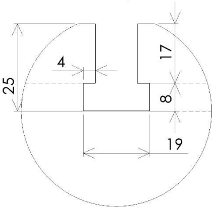
詳細図 B
