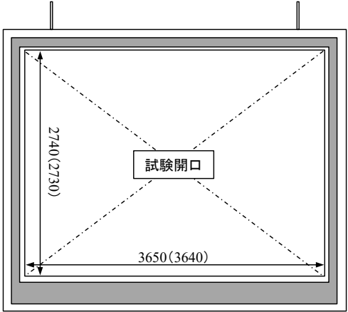
正面図 (( )内の数字は、試験体目安寸
