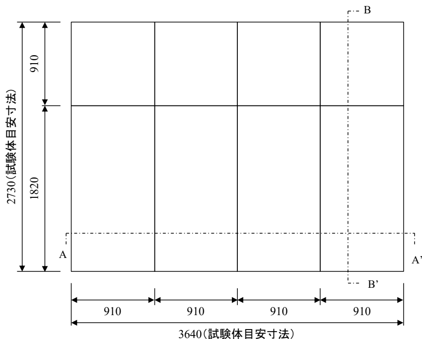
見本図 1 試験体配置図（単位：mm）
