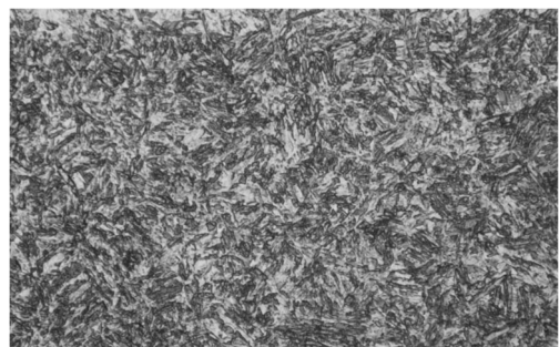
SCM440 マルテンサイト
