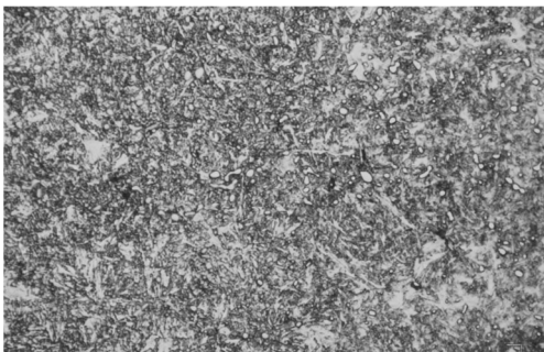
SKS93 マルテンサイト+球状セメンタイト
